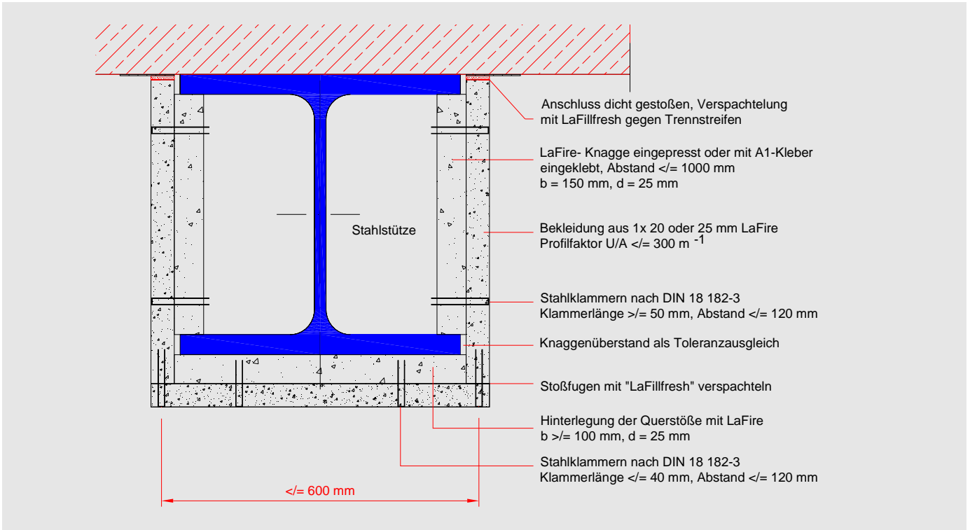
Bekleidung aus LaFire 20 und 25 mm
