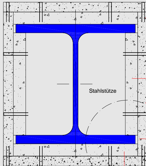
Schnitt Stoßfugenhinterlegung
