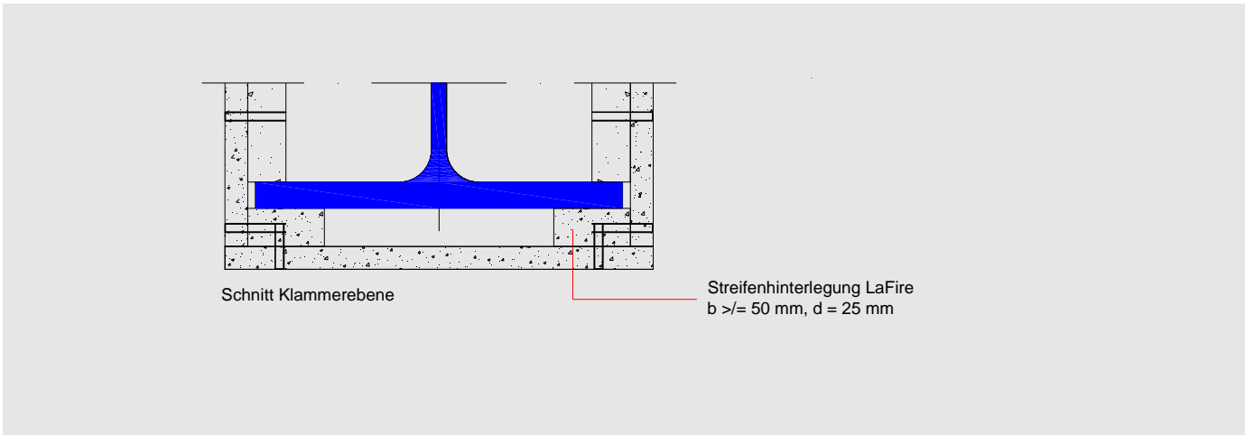
Bekleidung aus LaFire 15 mm; Schnitt Klammerebene
