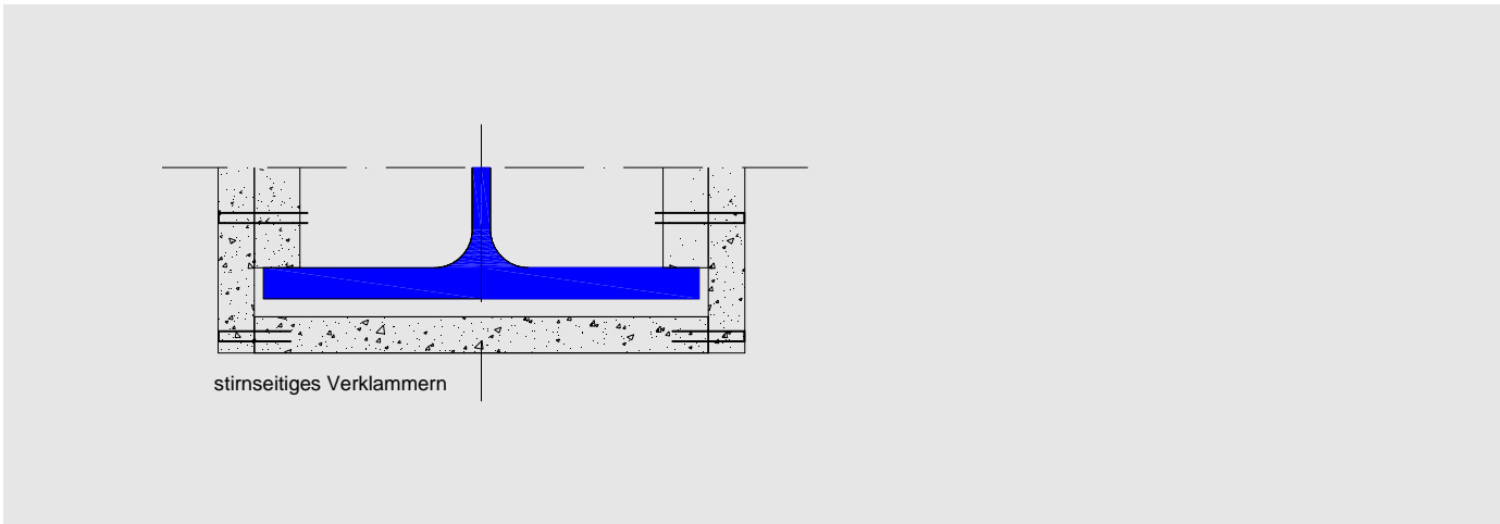
Variante; Flanschbekleidung zwischen die Seitenbekleidung geklammert
