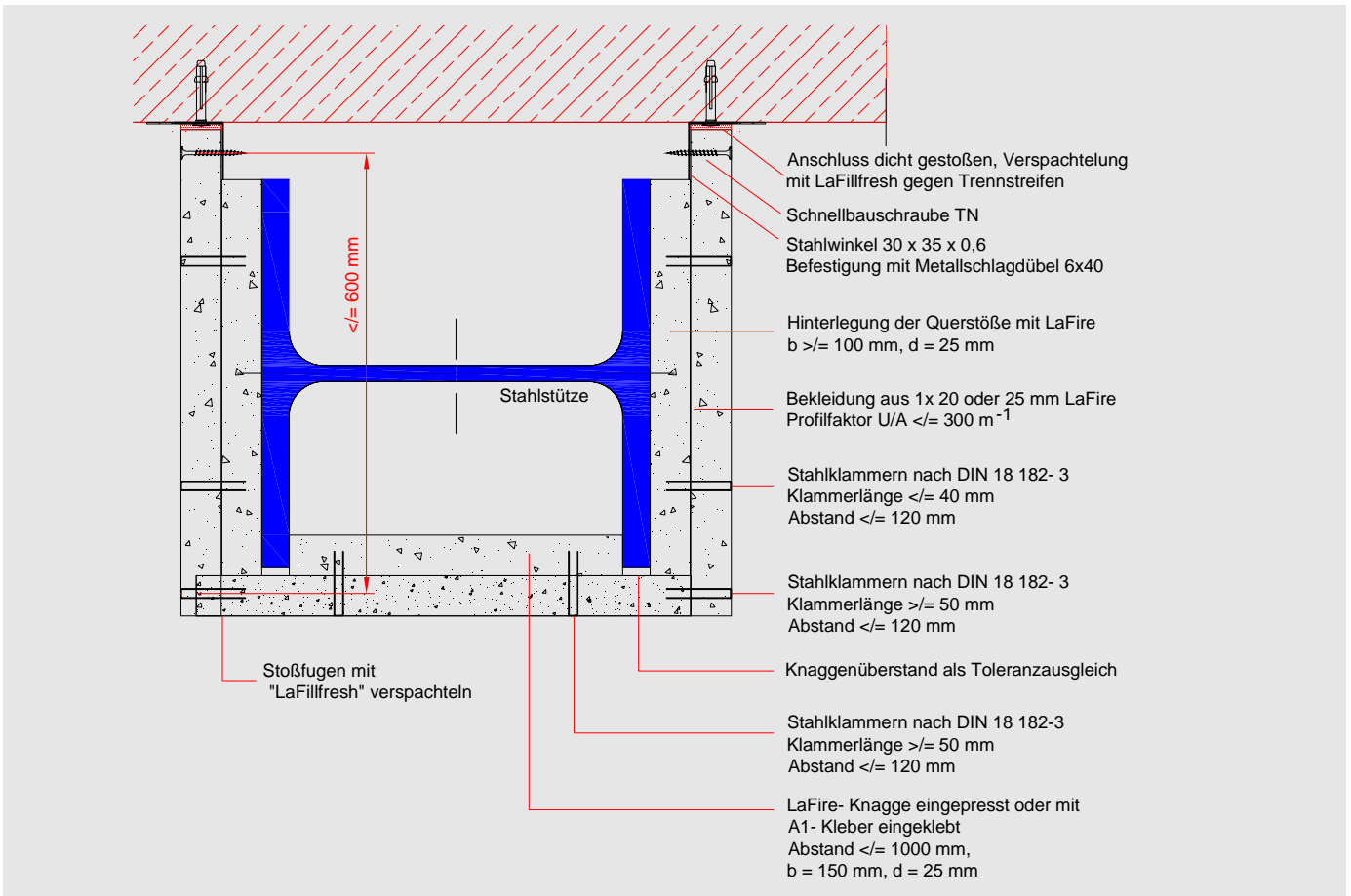
Bekleidung aus LaFire 20 oder 25 mm; Knagge LaFire und Blechwinkel
