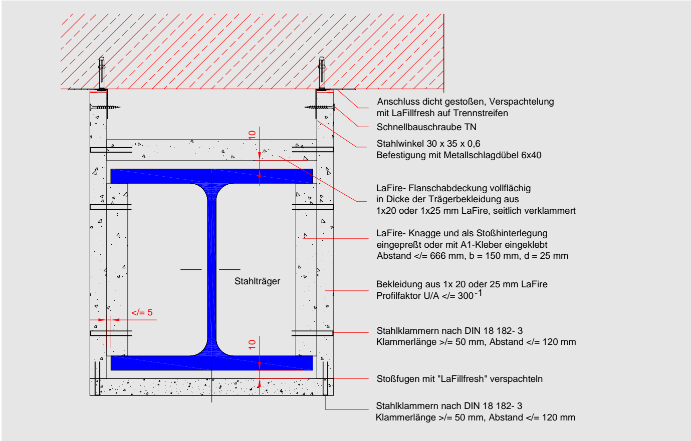
Bekleidung aus LaFire 20 oder 25 mm; Flanschbekleidung aufgesetzt
