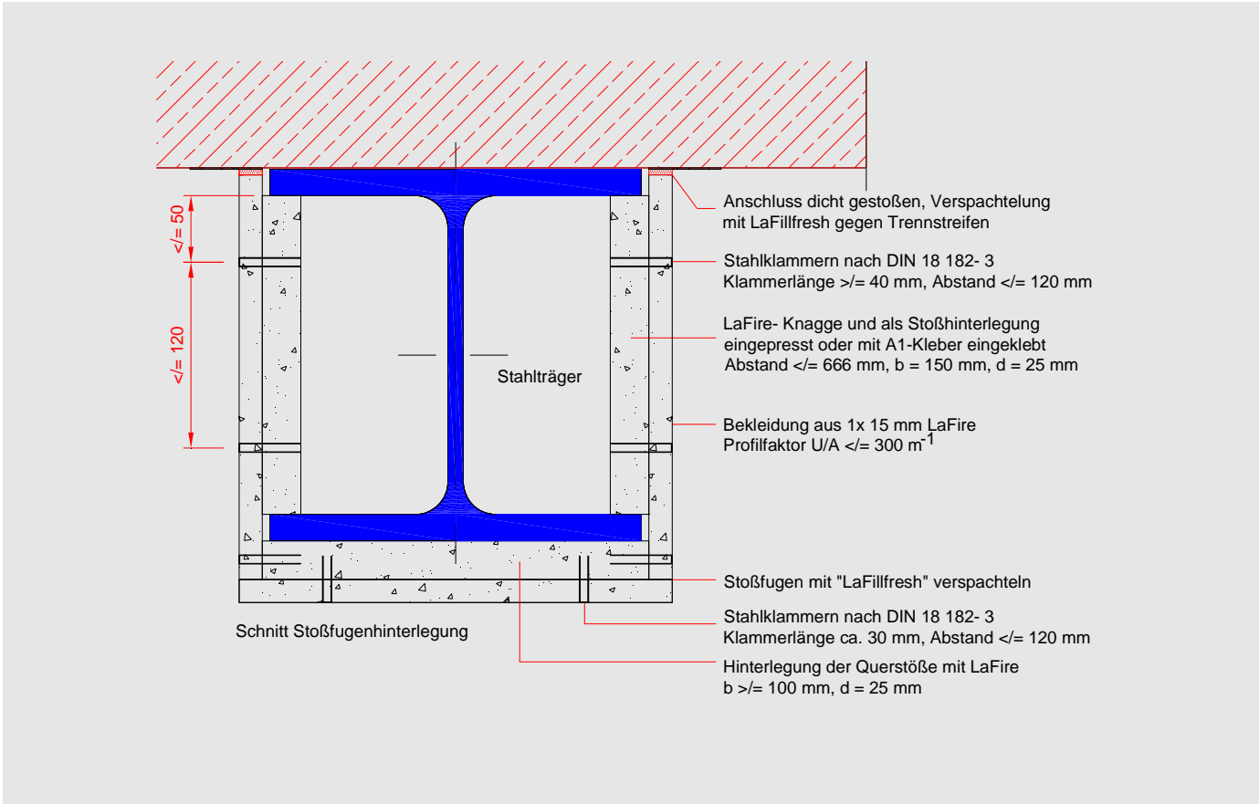
Bekleidung aus LaFire 15 mm; Schnitt Stoßfugenhinterlegung
