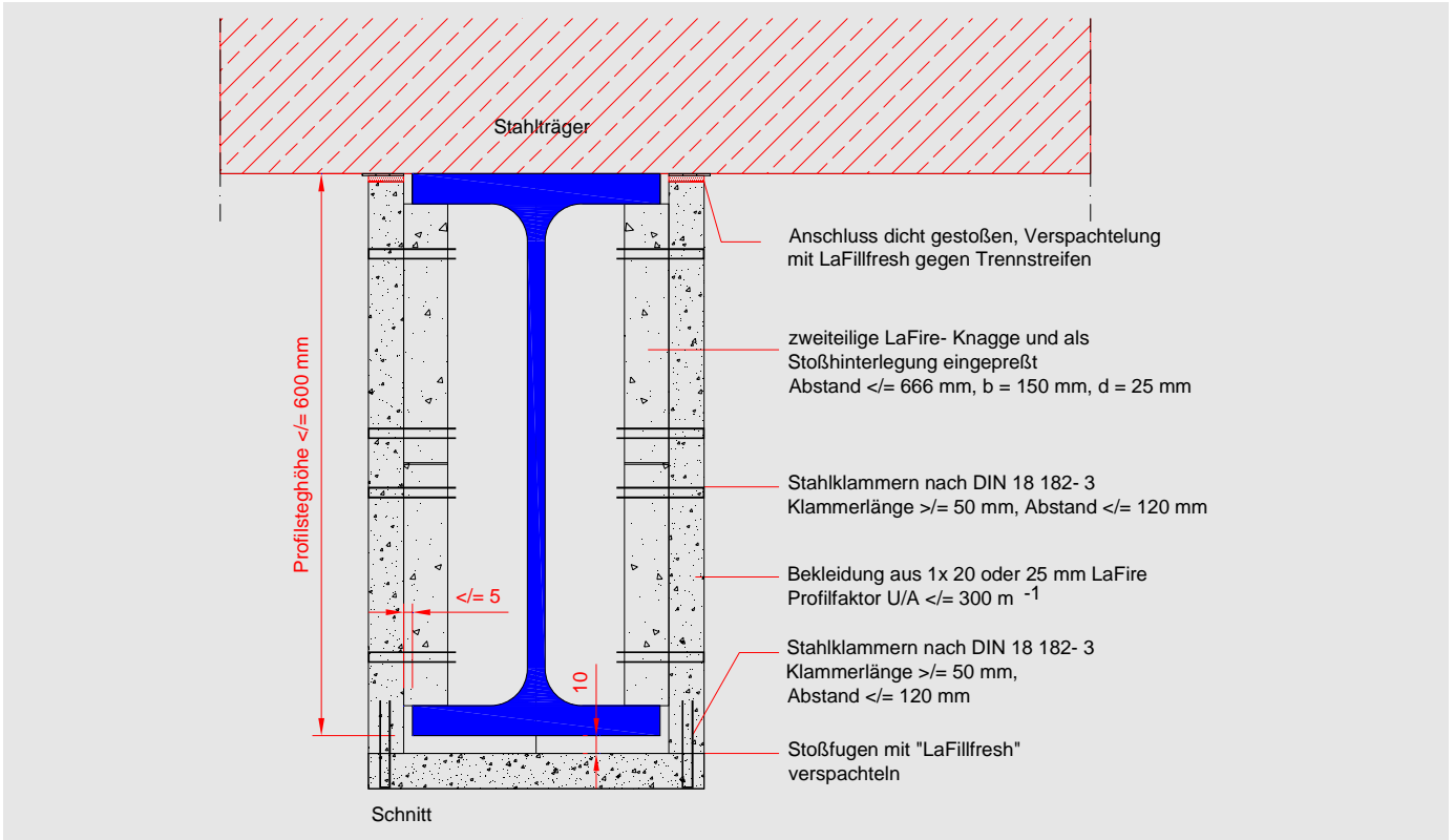
Bekleidung aus LaFire 20 oder 25 mm; zweiteilige Knagge
