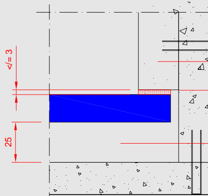
Schnitt Klammerebene
