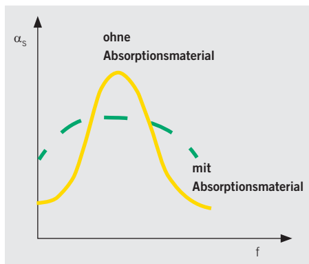
Schematische Darstellung: Absorptionsgrad eines Helmholtzresonators mit und ohne Hinterlegung (Vlies oder Mineralfaser)
