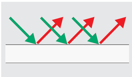
Vollständige Schallreflexion \alpha = 0 Glatte Oberfläche
