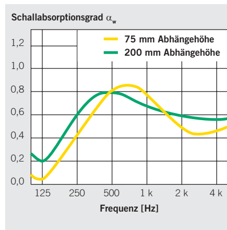
Absorptionskurven: Schallabsorptionsgrade von Lochplatten mit unterschiedlichen Abhängehöhen.
